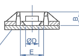
Sección B-B
